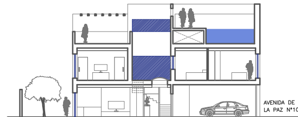
SECCIÓN LONGITUDINAL
