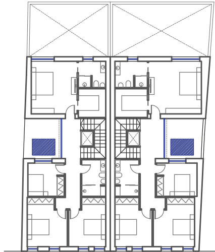
PLANTA ALTA
