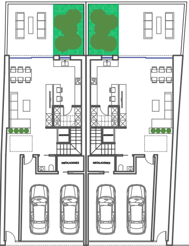
PLANTA BAJA
